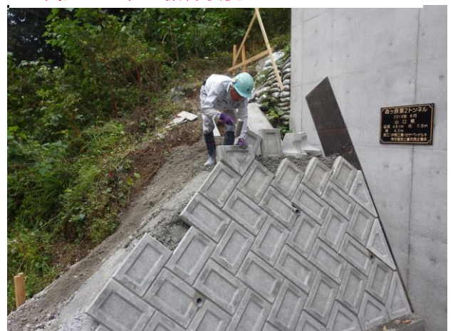
☆間知ブロック据付状況☆
